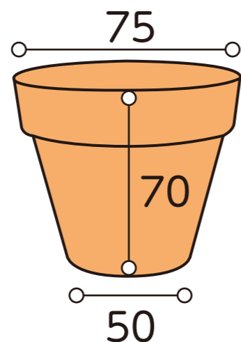
植木鉢 高さ70mm×上面φ75mm×底面φ50mm
