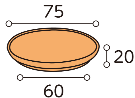
受け皿 高さ20mm×上面φ75mm×底面φ60mm
