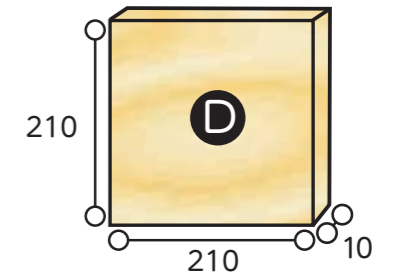
木材D (コ型用板) 約210×210×10mm×1枚
