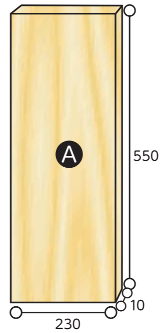
木材A (正面板) 約230×550×10mm×1枚
